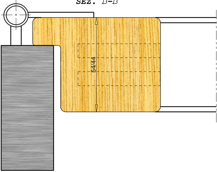
SEZ. B-B
