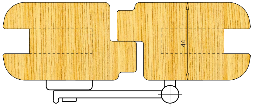
SEZ.C-C
