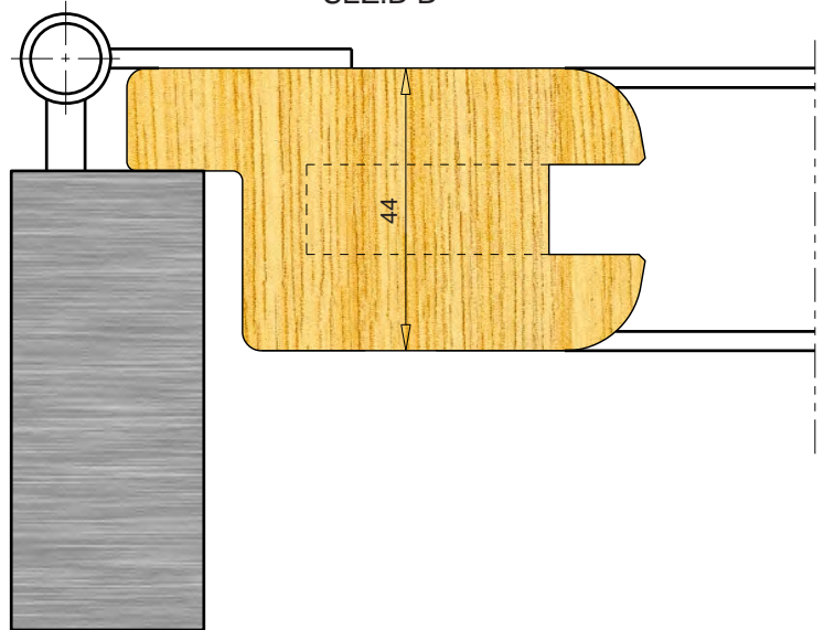
SEZ.B-B
