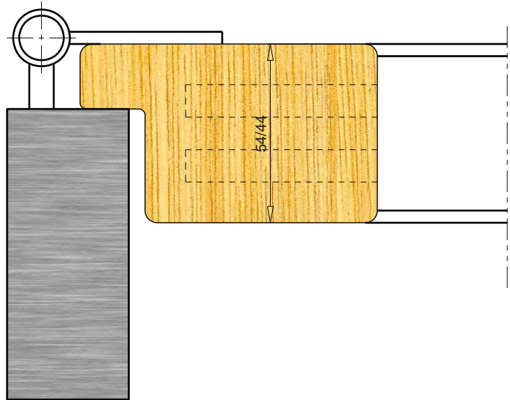
SEZ.B-B
