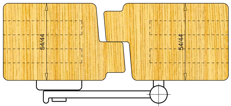
SEZ.C-C
