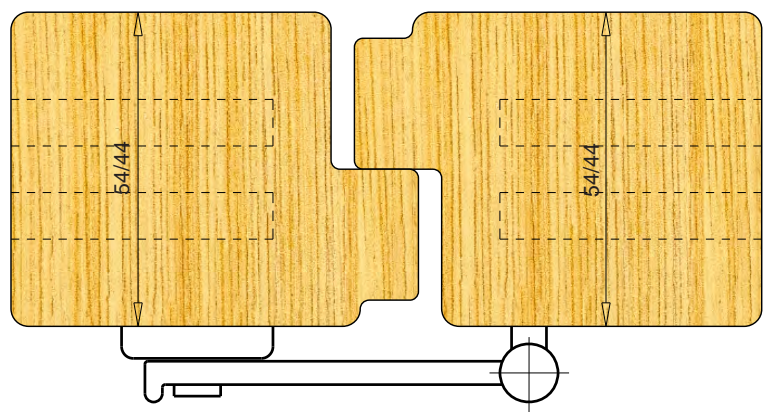
SEZ.C-C
