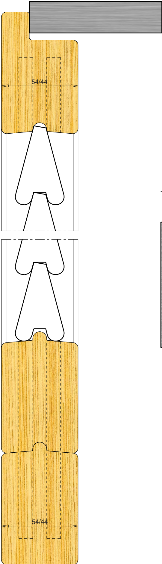
SEZ.A-A
